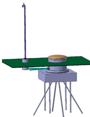
Concetto di installazione in campo libero
