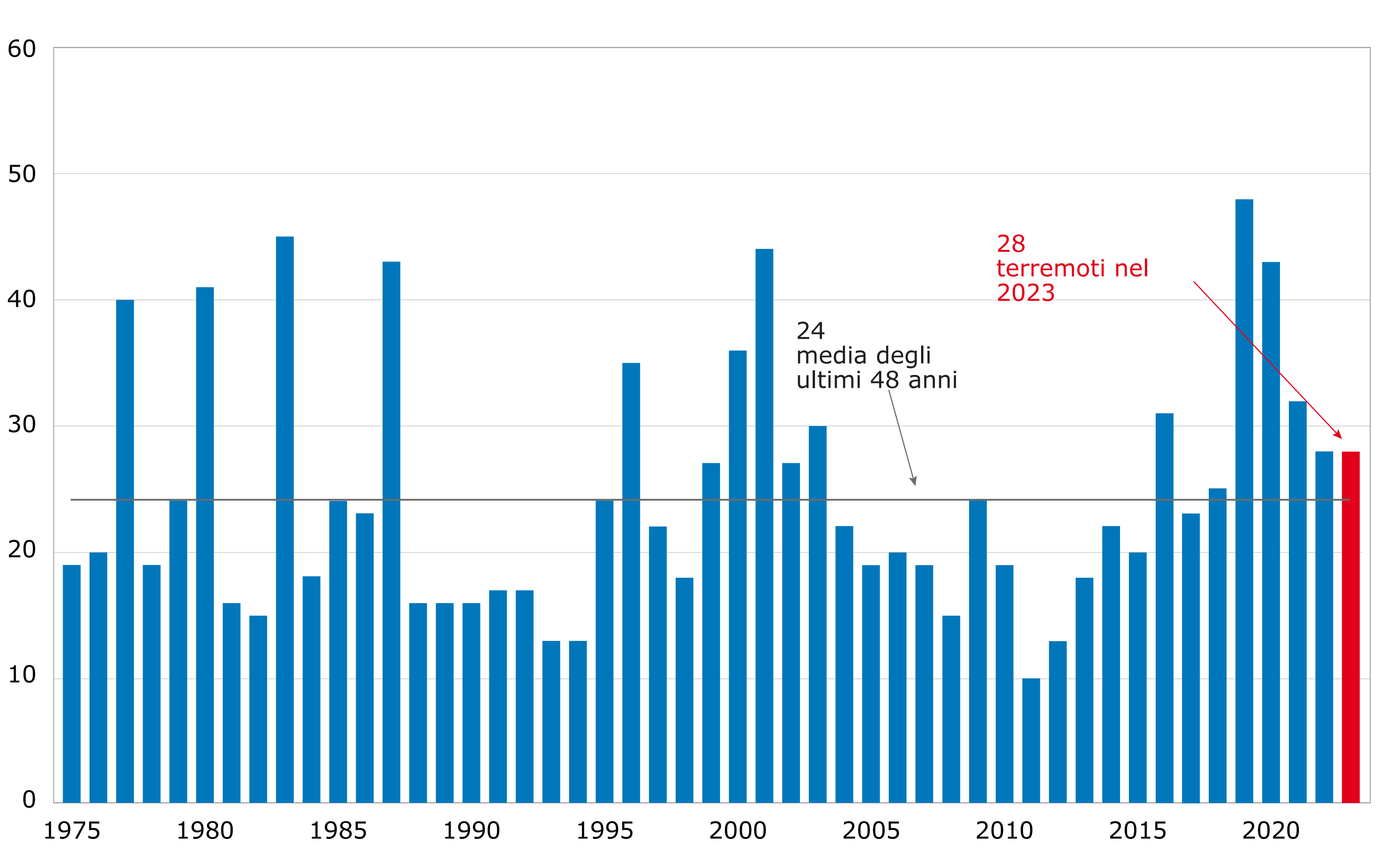
Numero di terremoti di magnitudo 2.5 o superiore per anno
