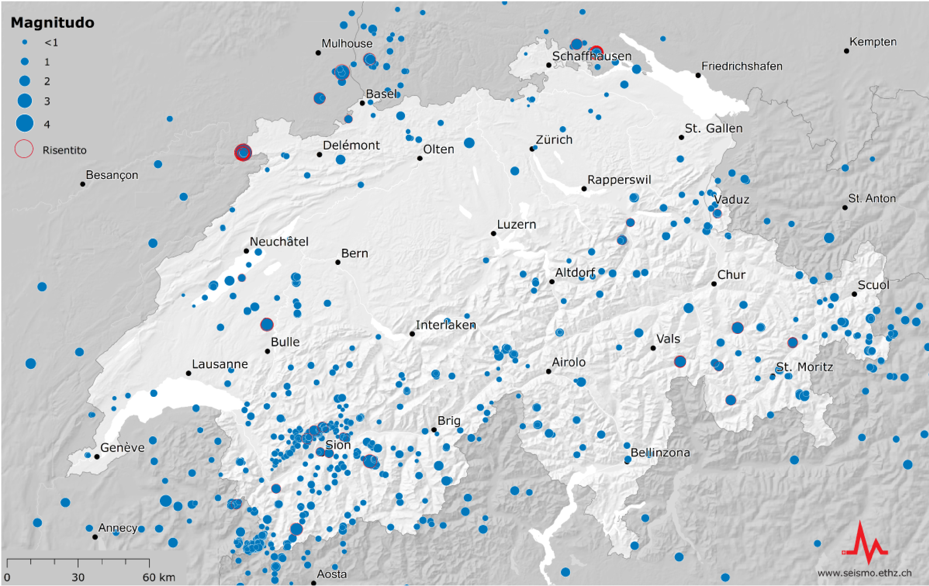
Tutti i terremoti registrati nel 2023
