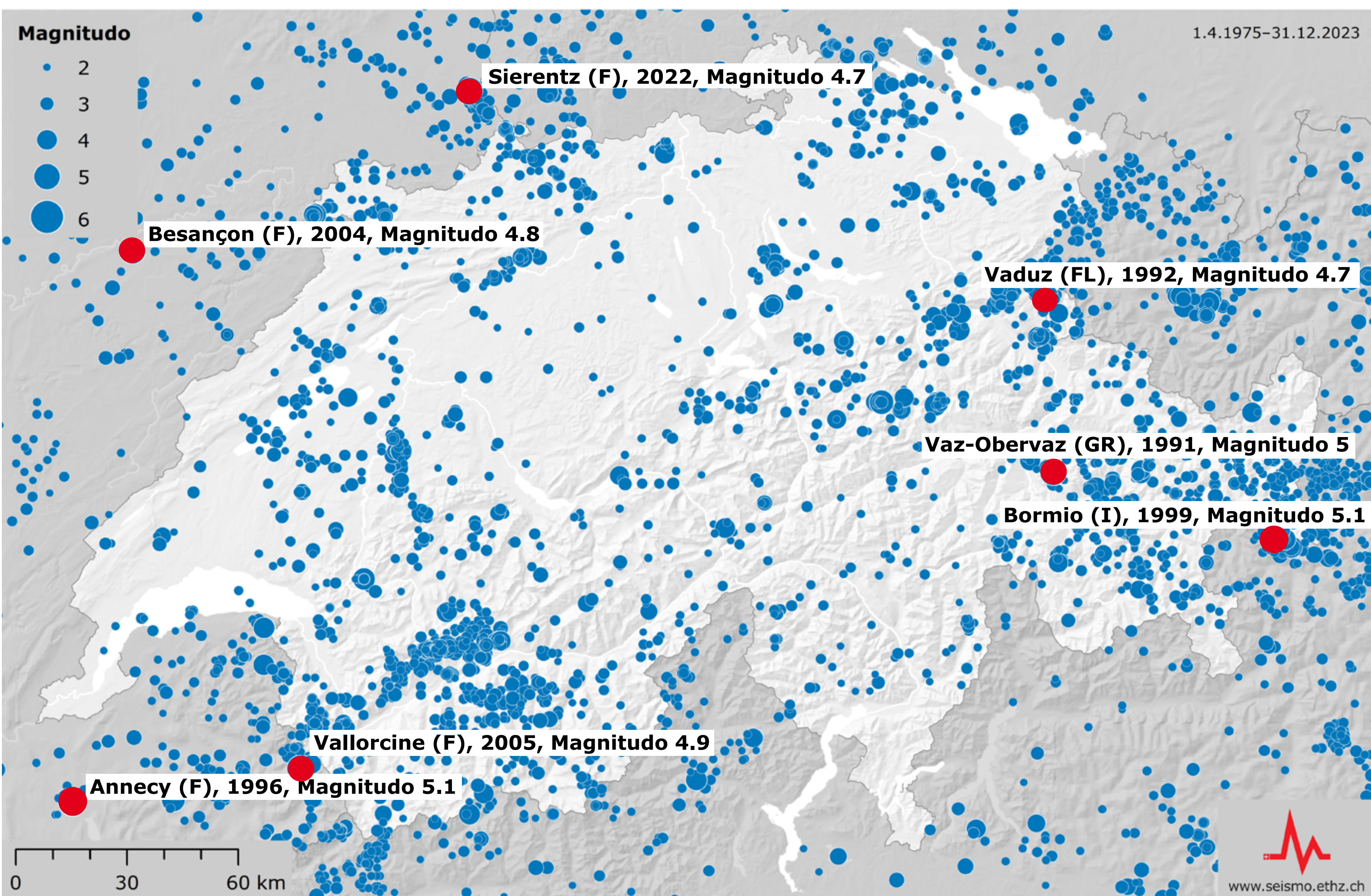
I terremoti più forti dal 1975
